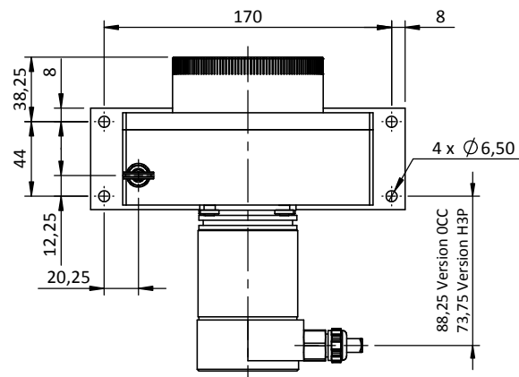
MHM5 - PROF/CANO/DNET Encoder Anschluss H3P oder OCC (Bushaube)
