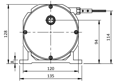
Anschluss C (Steckverbinder M16, 3-polig DIN)
