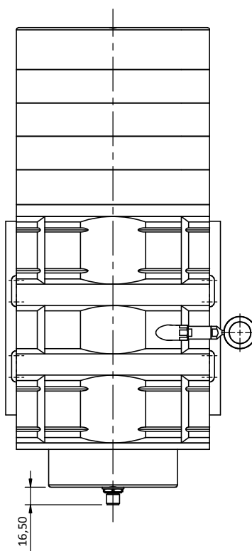
Anschluss L4 (Steckverbinder M12, 4-polig)
