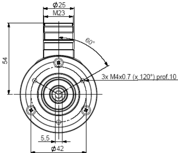
CHM5_06 Anschluss CPR / C1R (Stecker, M23, radial), mit Synchroflansch 9500/003 montiert*
