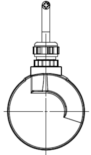
CHM5_06 Anschluss CPR / C1R (Stecker, M23, radial), mit Synchroflansch 9500/003 montiert*
