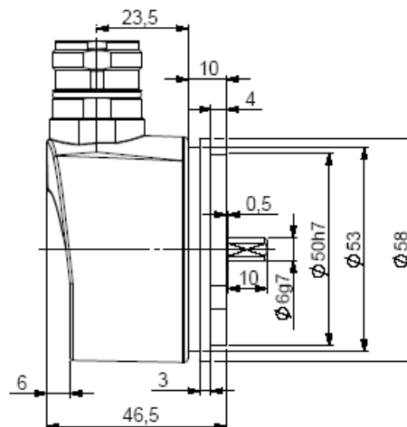
CHM5_06 Anschluss CPR / C1R (Stecker, M23, radial), mit Synchroflansch 9500/003 montiert*
